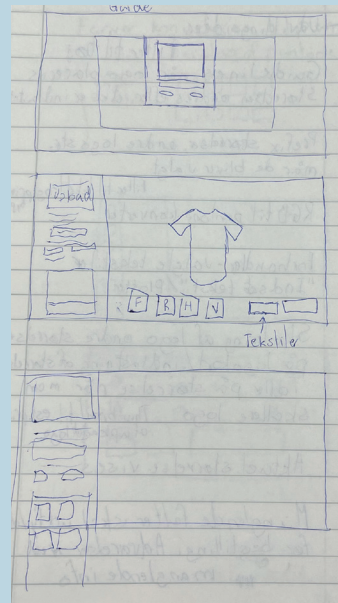
Web flow
